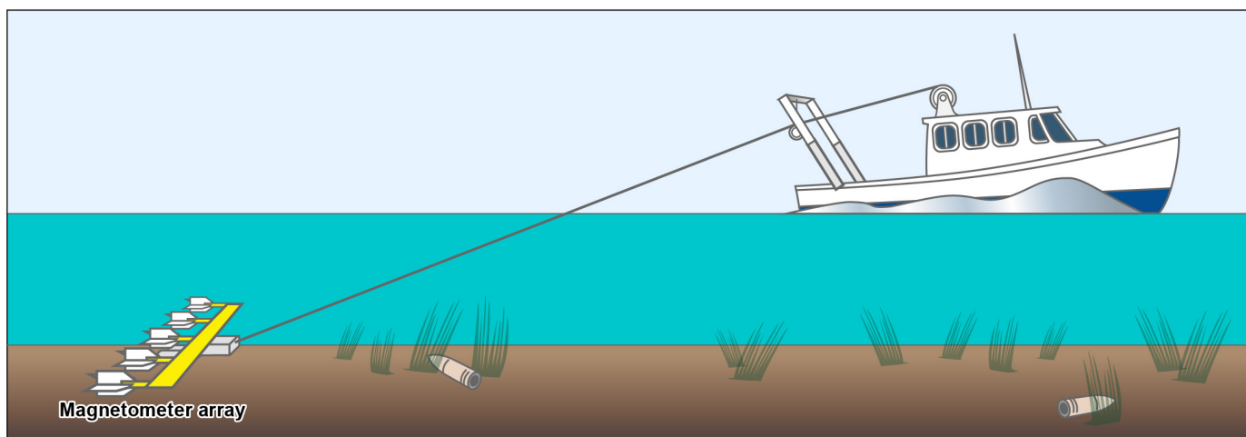
Figura 12: Tecnología del conjunto de magnetómetros remolcados que se usa en Vieques, Puerto Rico
